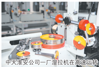
中天淮安公司一厂湿拉机在高速运转
