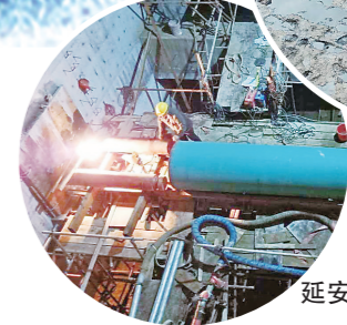
内城河铸铁管卡箍安装
